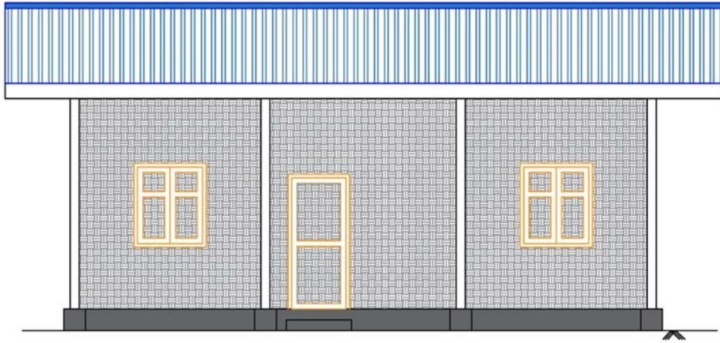
အနောက်ဘက်မှ မြင်ရသည့်ပုံစံ
