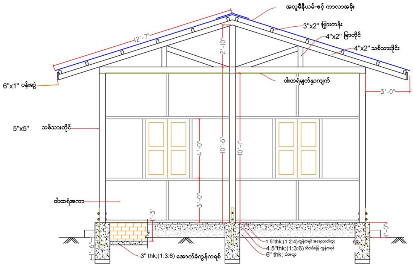
ကန့်လန့်ဖြတ်ပိုင်းပုံ
