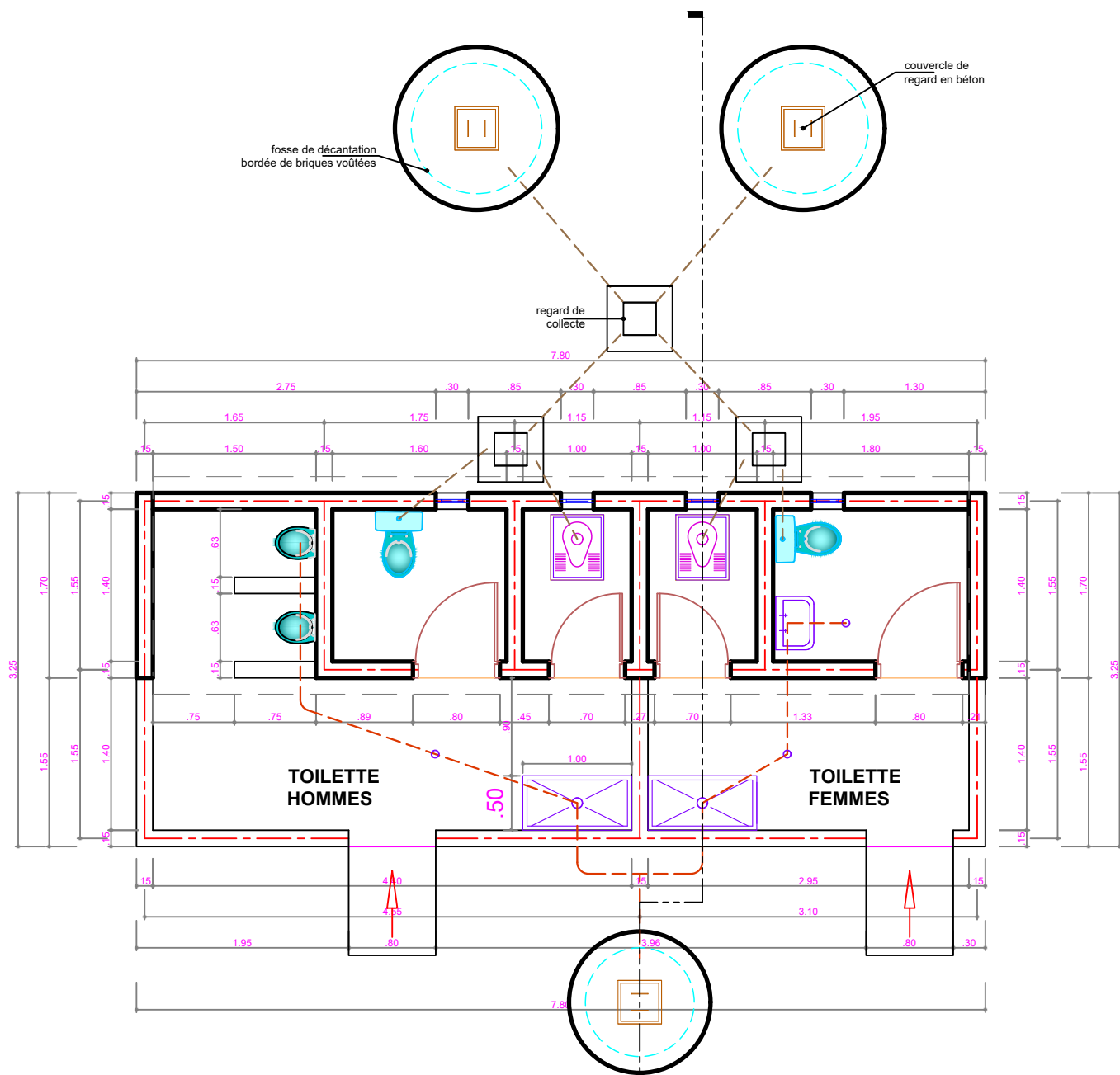
VUE EN PLAN REZ DE CHAUSSEE
