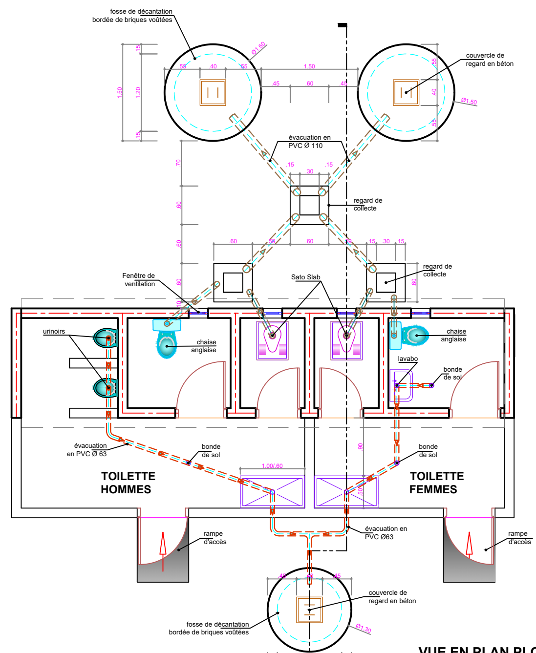
VUE EN PLAN PLOMBERIE
