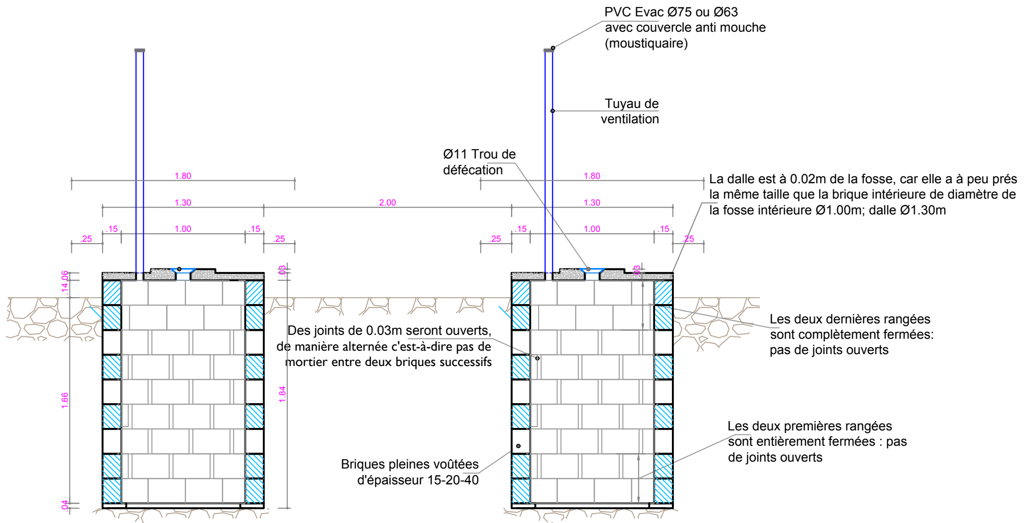
COUPE AA
