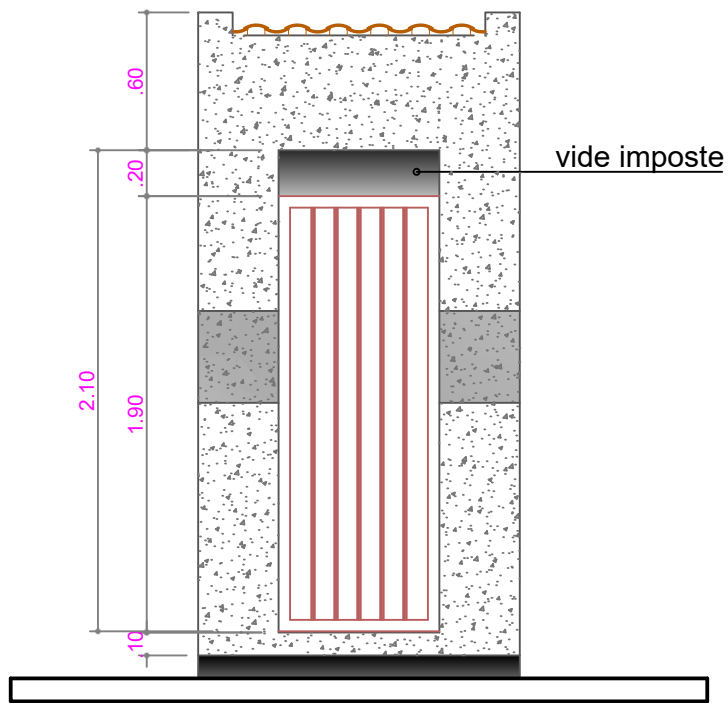
FACADE PRINCIPALE
