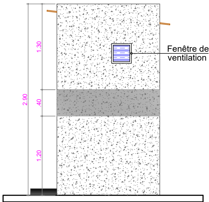
FACADE LATERALE DROITE
