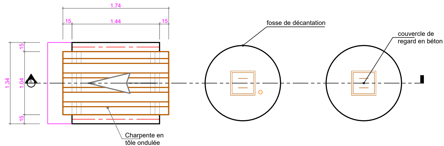
VUE EN PLAN TOITURE
